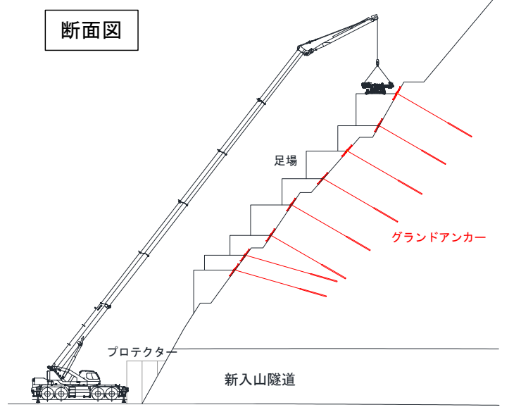
新入山隧道坑口部 法面補強工
